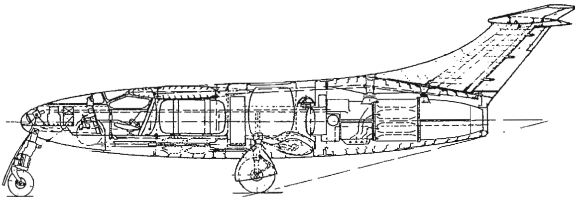
Messerschmitt Zerstörer Scheme I sectional side-view.
