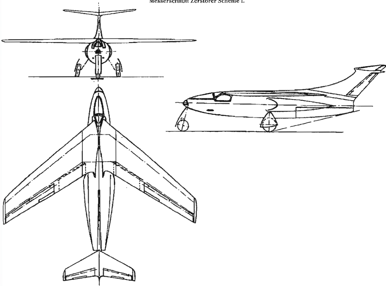
Messerschmitt Zerstörer Scheme I.
