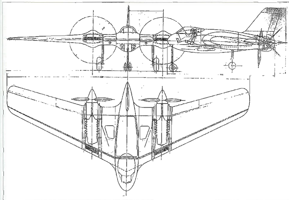
Messerschmitt Me 329.
