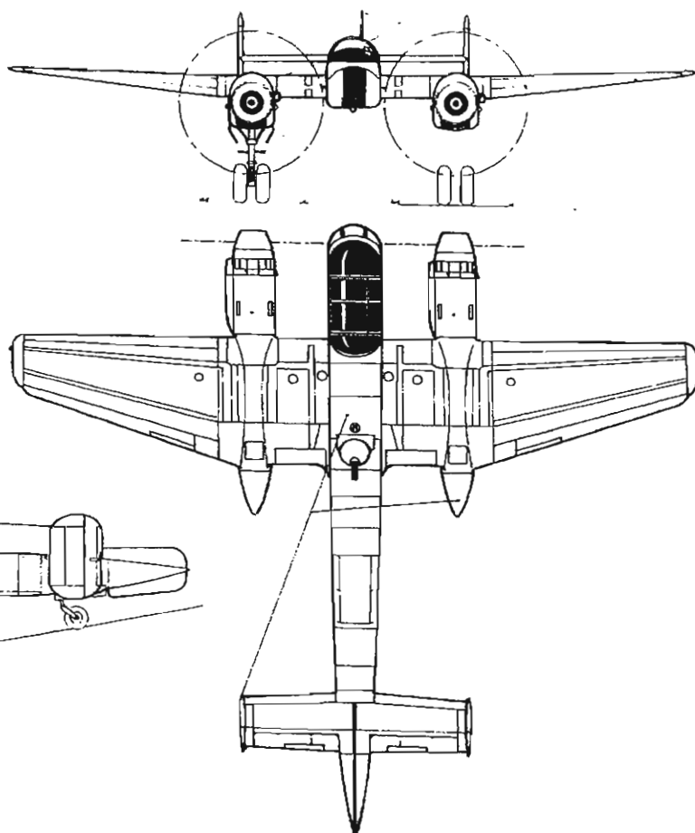
Arado Ar 240A-01.
