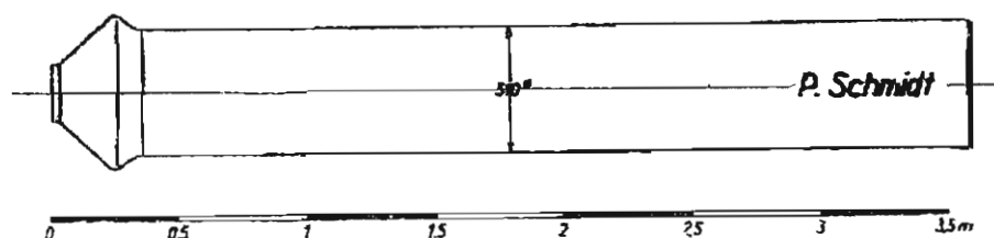
The Paul Schmidt SR 500 pulsejet.
