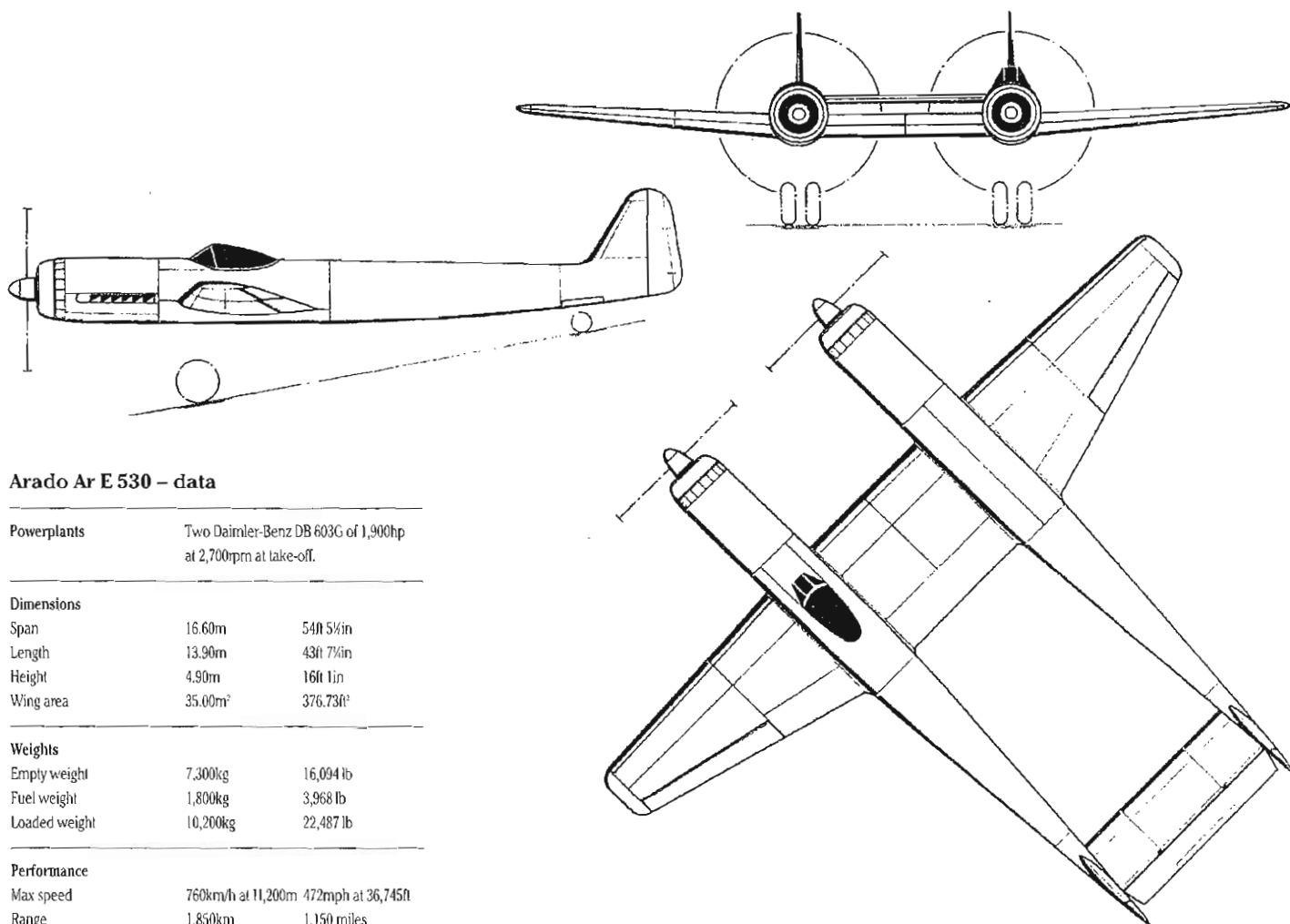
Arado E 530.
