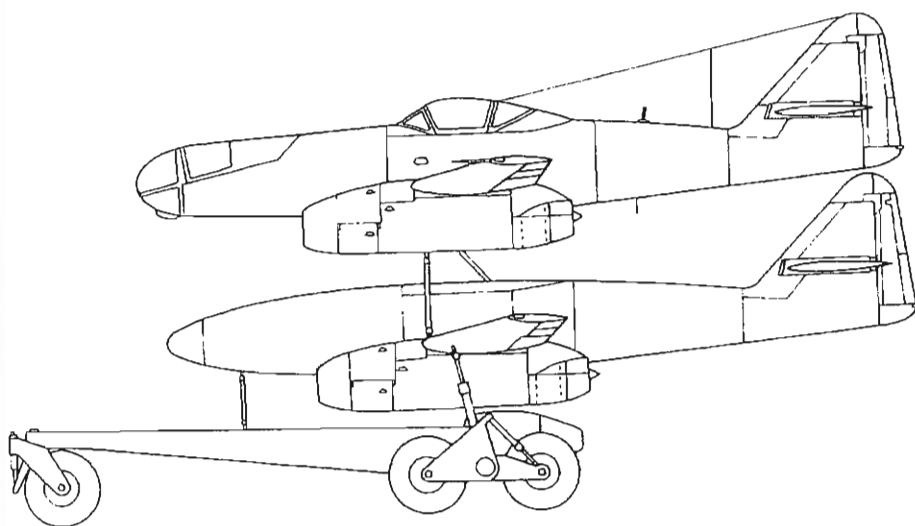
Messerschmitt Me 262A-2/U2 + Me 262A-1 'Mistel' composite.
