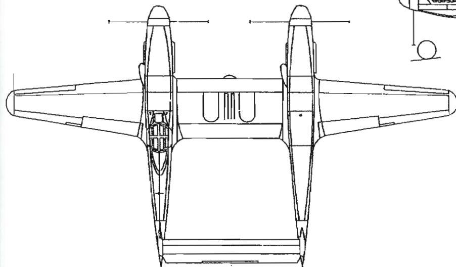
Messerschmitt Me 609.
