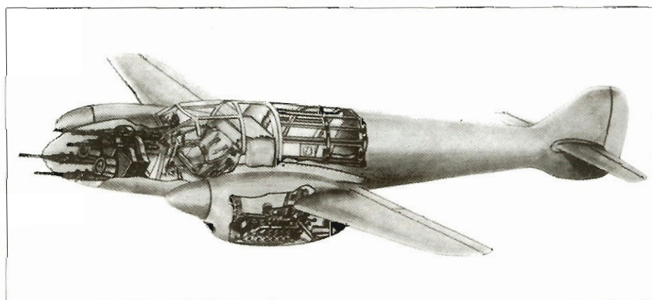
Top: Gotha P 20.
