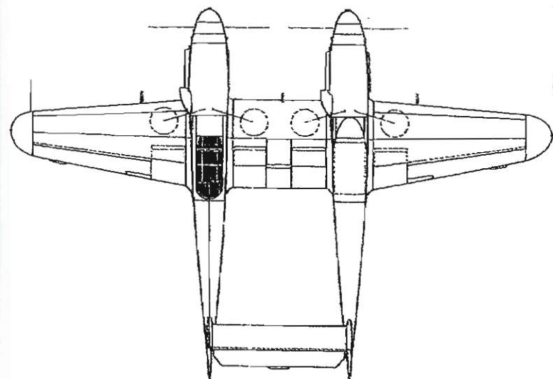
Messerschmitt Me 109Z.
