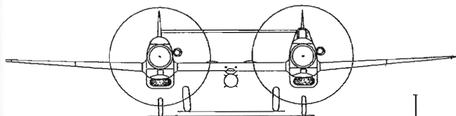
Messerschmitt Me 609.
