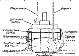
Vergleich zwischen Fliegerbombe u. Granate von gleichem Gewicht
