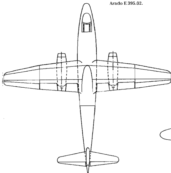
Arado E 395.02.
